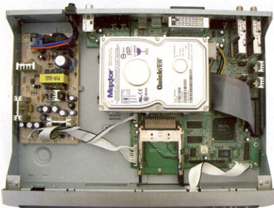
Das Innenleben des PVR-5020
